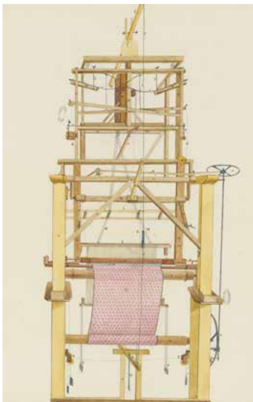
Dessin d'un métier à tisser dans un dossier de demande de brevet d'invention, par Tournu et Martinon. 1810. Archives nationales, F/12/1044.
